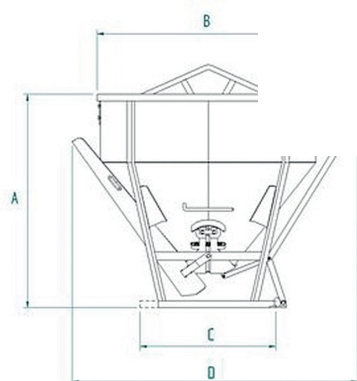
Benne conique à fond ouvrant avec goulottes latérales
